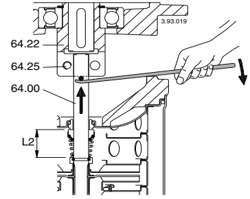
Fig. 6b Rotor elevado, posición de bloqueo del eje en el manguito.
