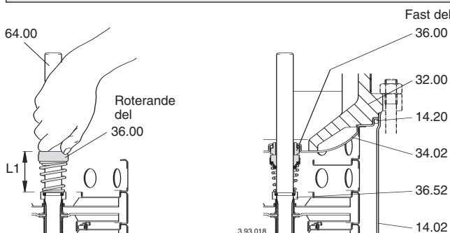
Fig. 5 Montering av axeltätning
