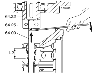
Abb. 6b Angehobener Läufer, Blockierposition Welle in Kupplung.
